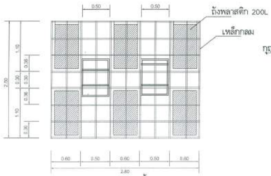
แบบแปลนหน้า
