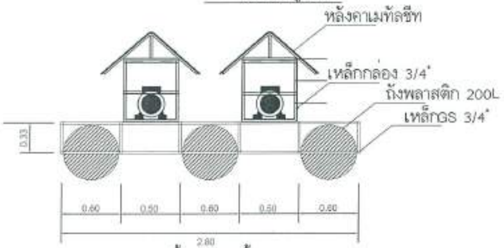
รูปด้านแปลนหน้า
