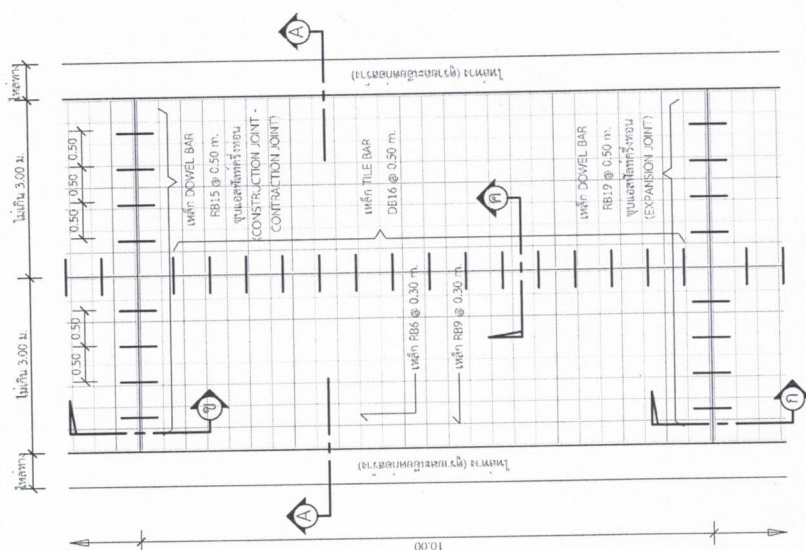
แปลนพนณน
